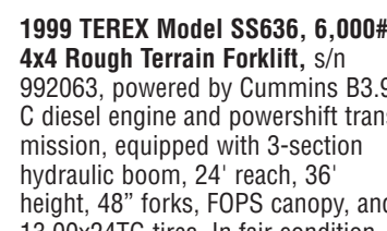
'99 TEREX 6,000#, 4X4
